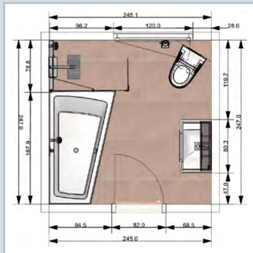
Grundriss
