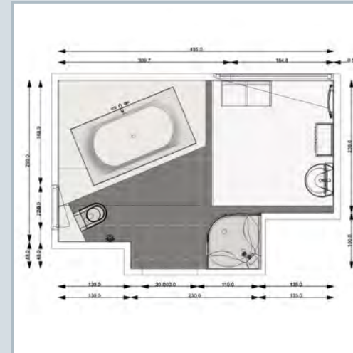
Grundriss
