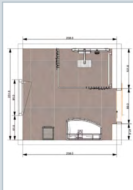
Grundriss
