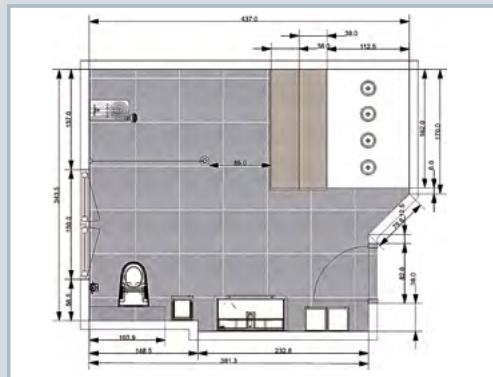
Grundriss
