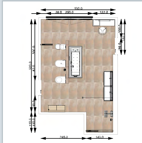
Grundriss
